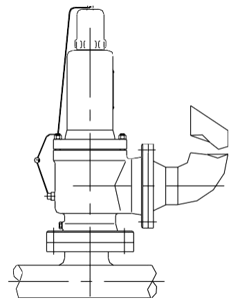
图3 用于空气、气体或蒸汽
